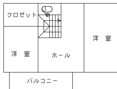
2F排水平面図
